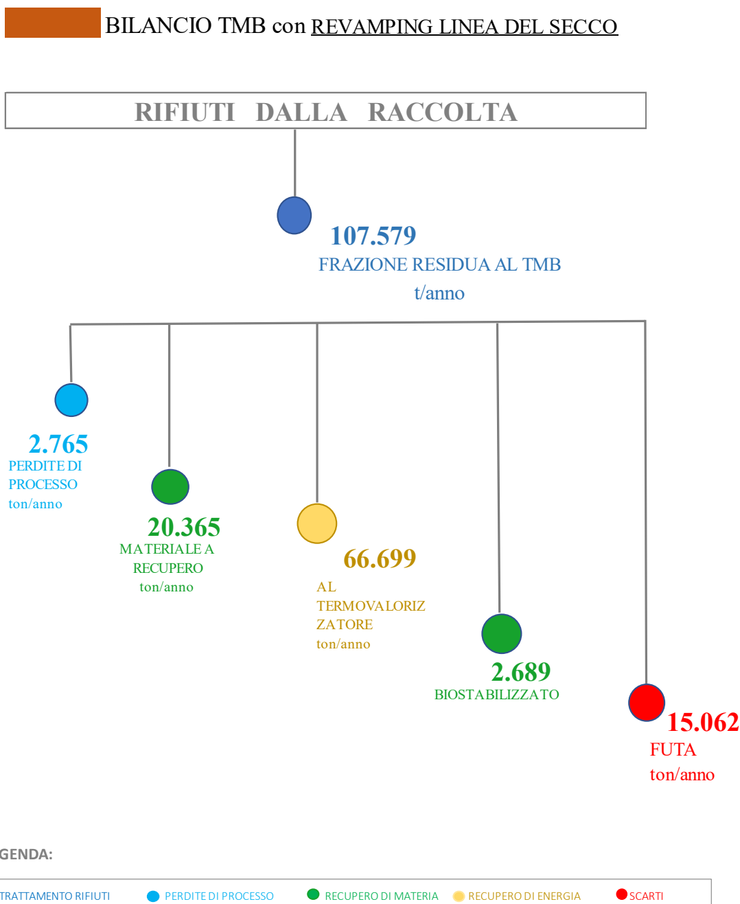
Figura 54: Bilancio TMB con revamping linea del secco (FST)
